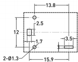
安装孔尺寸
